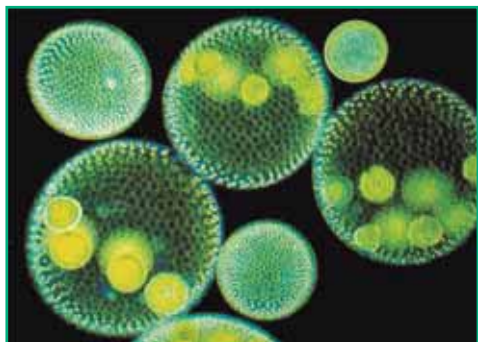
Рис. 69. Вольвокс
