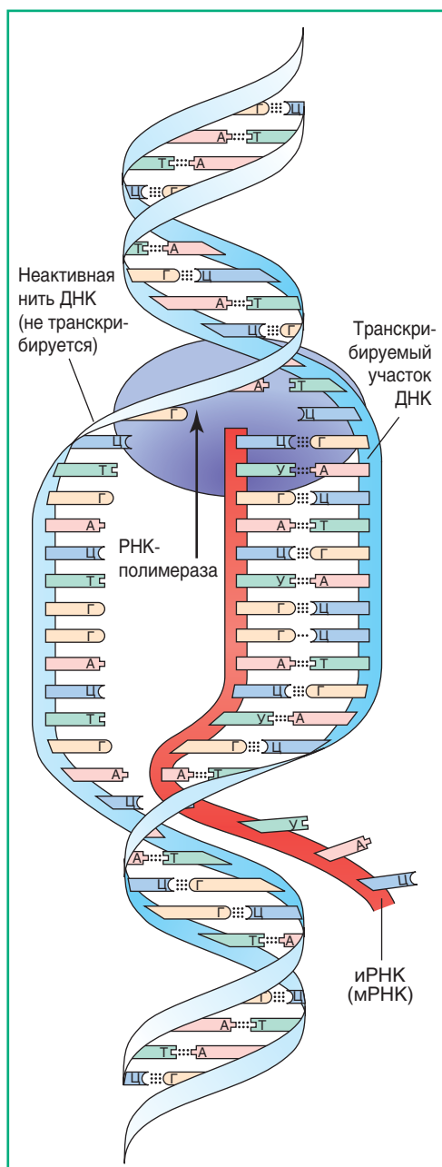
Рис. 65. Схема транскрипции
